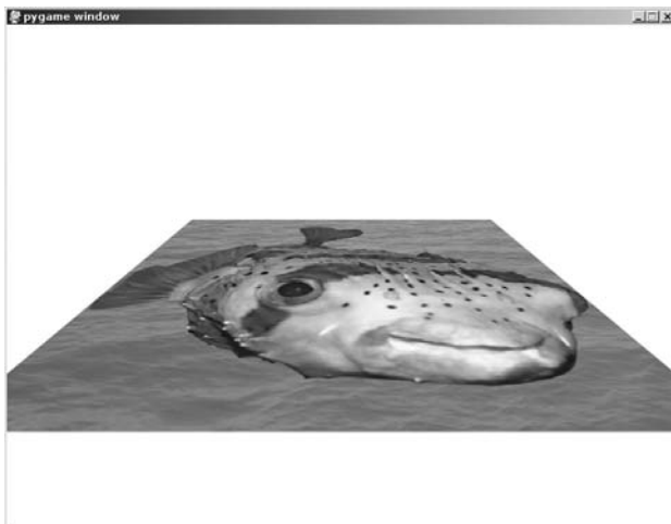
Figure 11-2. opengltext.py
