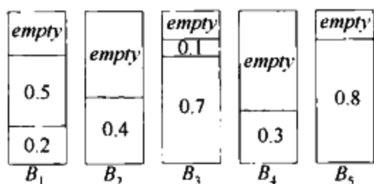
图 10-21 对 0.2, 0.5, 0.4, 0.7, 0.1, 0.3, 0.8 的下项适合算法
