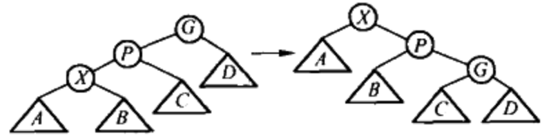
图 4-45 一字形(zig-zig)情形
