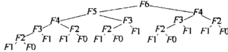
图 10-42 跟踪斐波那契数的递归计算
