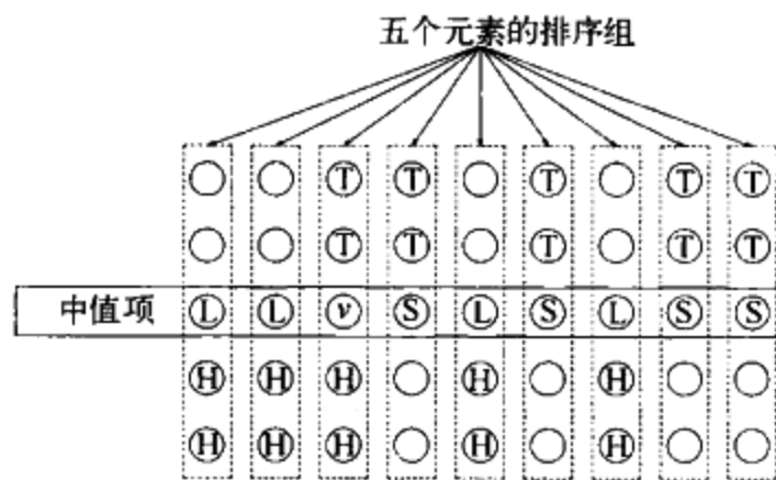
图 10-36 枢纽元的选择
