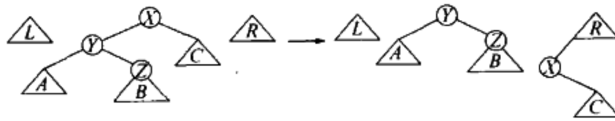
图 12-2 简化的自顶向下的之字形旋转
