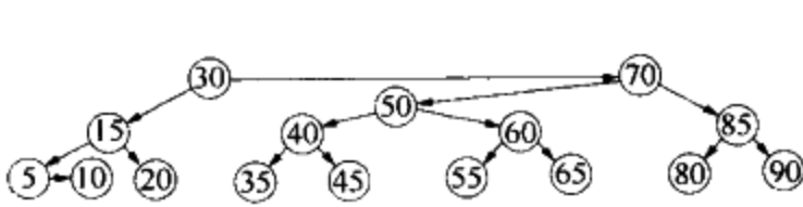
图 12-34 在 40 处 split 之后
