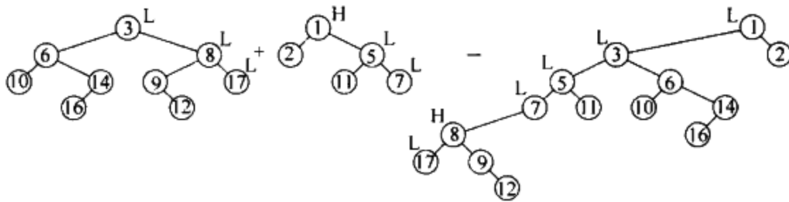
图 11-8 合并后重/轻状态的变化
