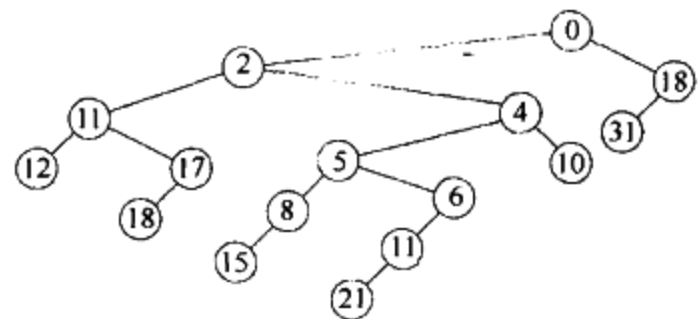
图 11-14 通过合并 H_1 和 H_2 而完成操作 decreaseKey( X, 9 )
