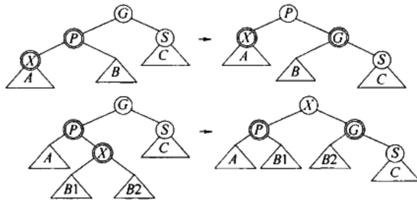
图 12-10 如果 S 是黑色的，则单旋转和之字形旋转有效
