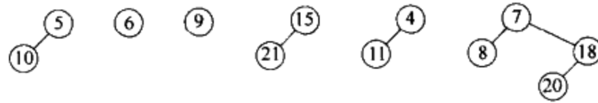
图 11-16 在删除最小元素(3)后的懒惰二项队列
