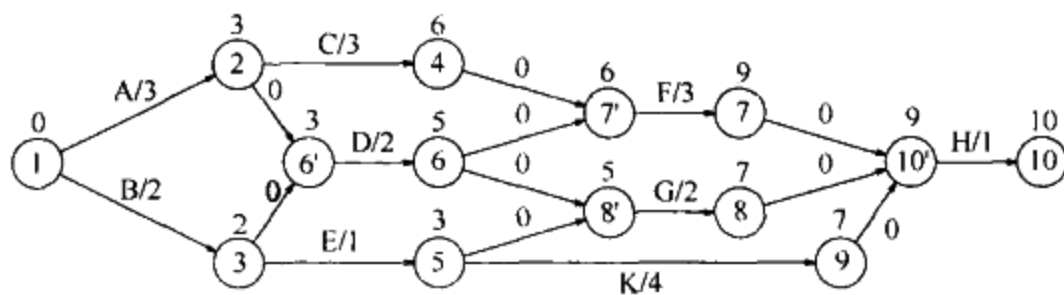
图 9-35 最早完成时间
