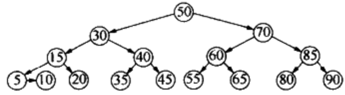
图 12-35 在 70 进行 skew 和在 30 进行 split 后最后得到的树
