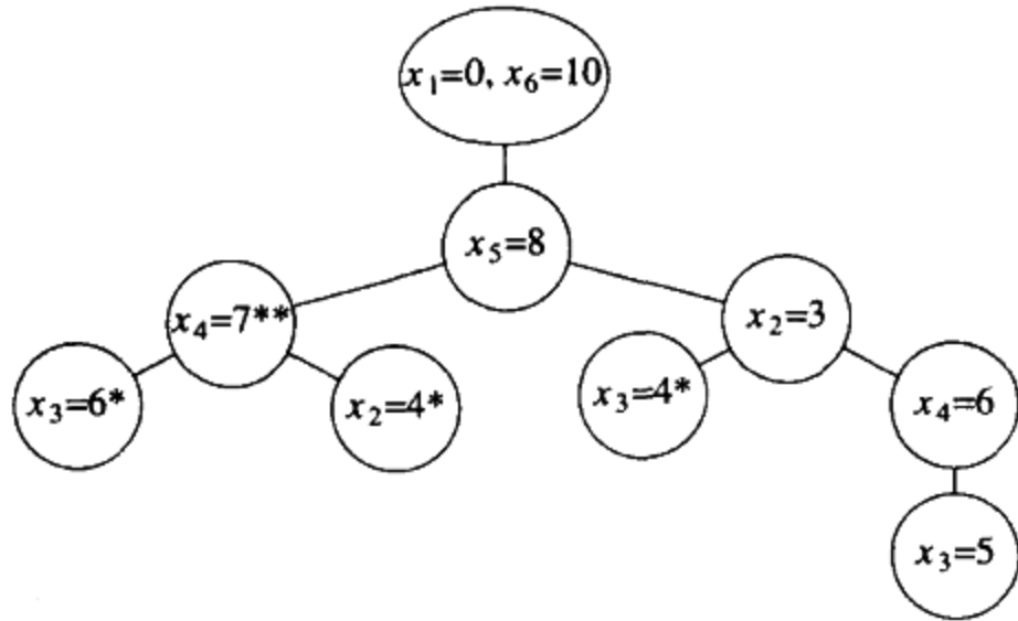
图 10-63 收费公路重建问题的决策树
