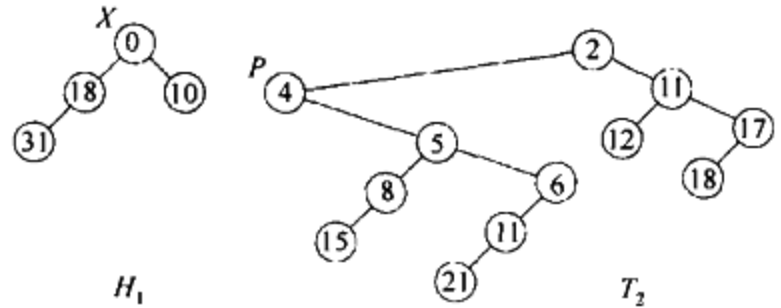
图 11-12 切断之后得到的两棵树
