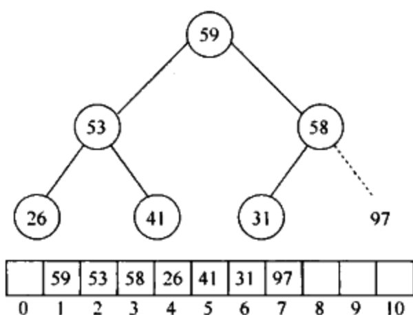
图 7-7 在第一次 deleteMax 后的堆
