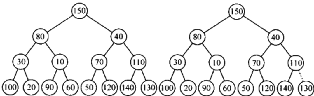
图 6-15 左: 初始堆; 右: 在 percolateDown(7)后
