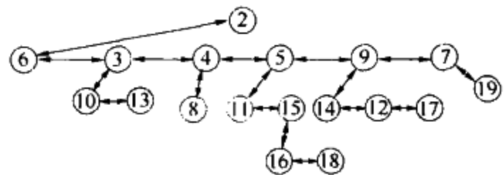
图 12-46 左面的配对堆的具体表示
