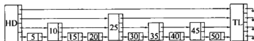
图 12-20 插入 27：其次，通过提升 35 将含 3 个高度为 1 的节点的间隙分裂
