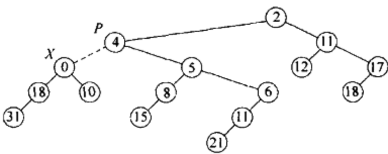
图 11-11 将 9 降到 0 引起堆序的破坏
