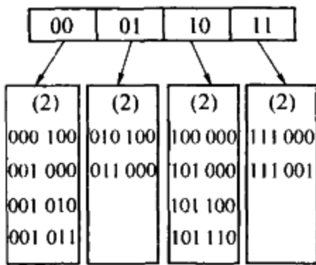
图 5-24 可扩散列: 原始数据
