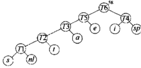
图 10-19 最后一次合并后的哈夫曼算法
