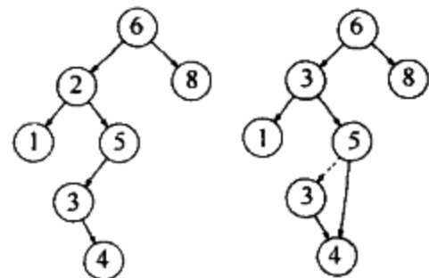
图 4-24 删除具有两个儿子的节点 2 前后的情况
