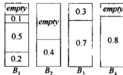
图 10-26 对 0.2, 0.5, 0.4, 0.7, 0.1, 0.3, 0.8 的最佳适合算法
