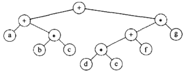
图 4-14 (a+b*c) + ((d*e+f)*g) 的表达式树
