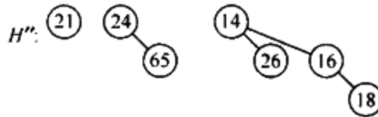
图 6-48 二项队列 H'' ：除去 12 后的 B_3
