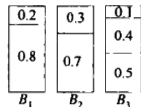
图 10-27 对 0.8, 0.7, 0.5, 0.4, 0.3, 0.2, 0.1 的首次适合算法
