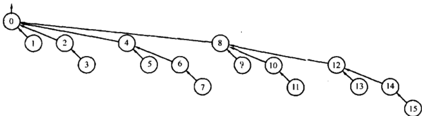
图 8-12 N = 16 时最坏情形的树
