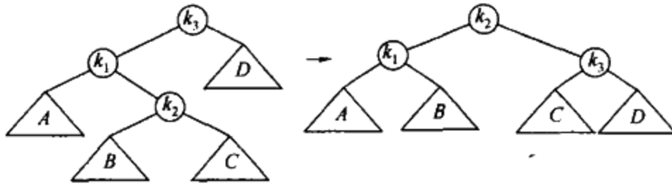
图 4-42 双旋转
