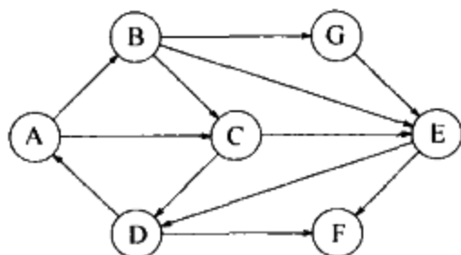
图 9-84 练习 9.26 中所使用的图
