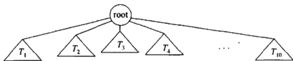
图 4-1 一般的树
