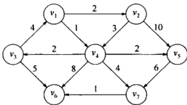
图 9-20 有向图 G
