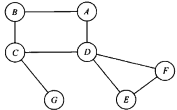
图 9-62 具有割点 C 和 D 的图
