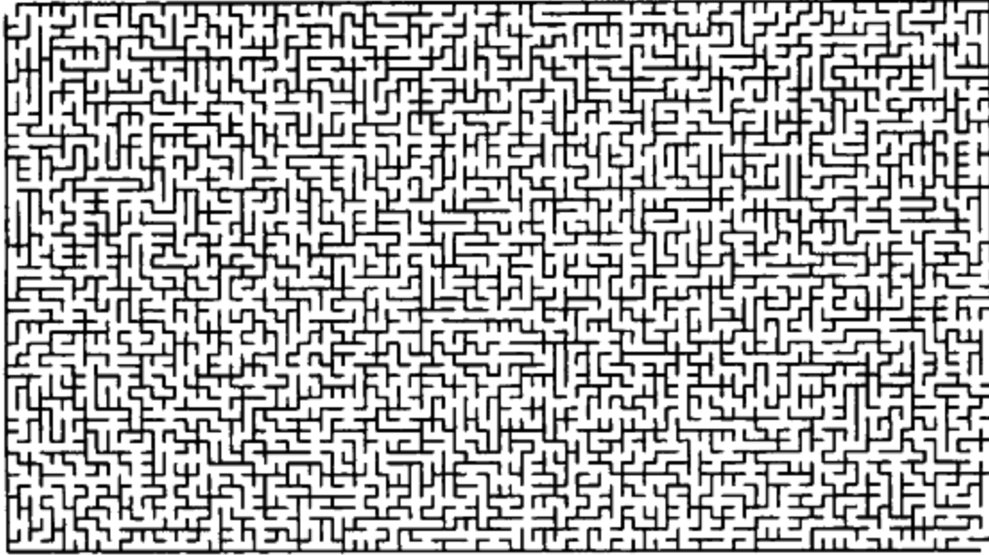
图 8-19 一个 50×88 迷宫
