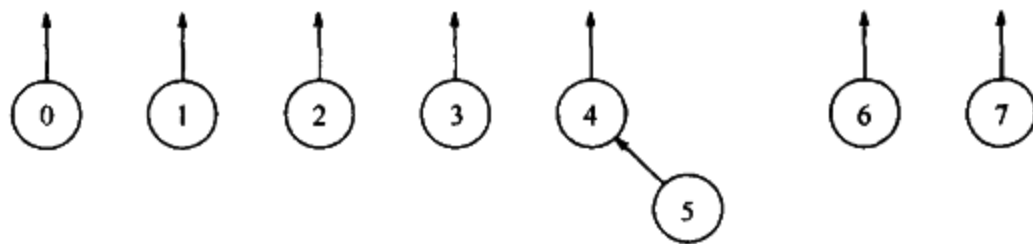
图 8-2 在 union(4, 5) 之后
