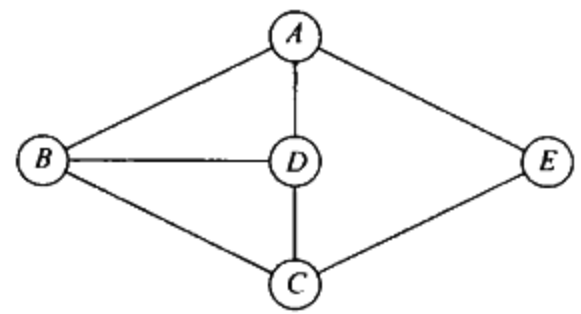
图 9-60 一个无向图
