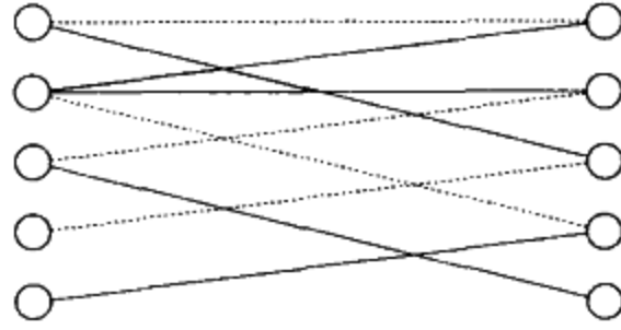
图 9-81 一个二分图
