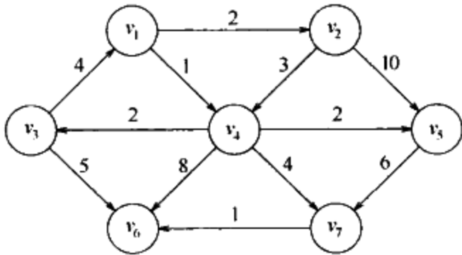
图 9-8 有向图 G
