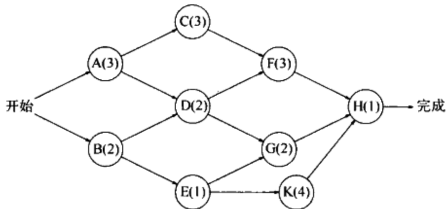
图 9-33 动作节点图
