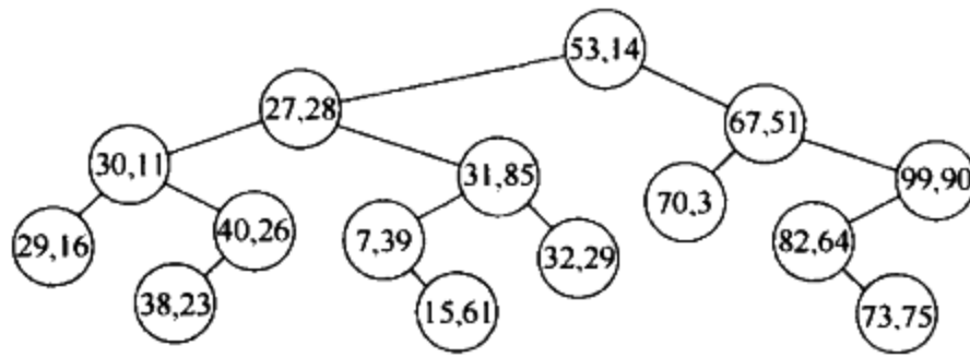
图 12-42 2- d 树示例
