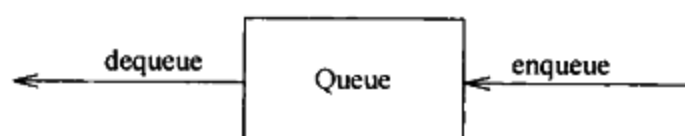
图 3-37 队列模型
