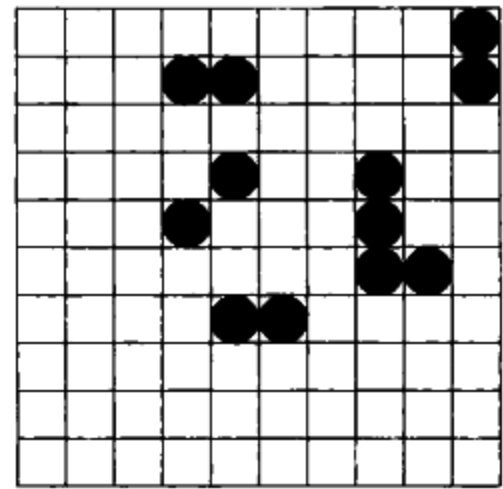
图 9-86 练习 9.45 中的网格
