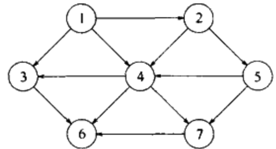
图 9-1 一个有向图
