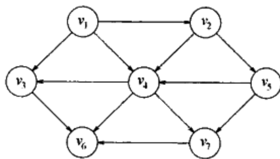
图 9-4 一个无圈图
