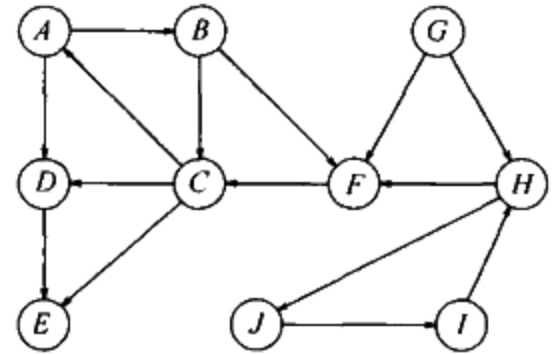
图 9-74 一个有向图
