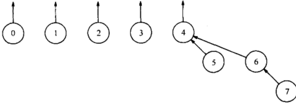
图 8-4 在 union(4, 6)之后
