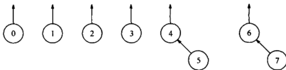
图 8-3 在 union(6, 7) 之后
