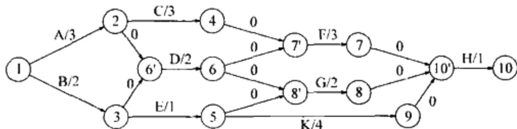
图 9-34 事件节点图
