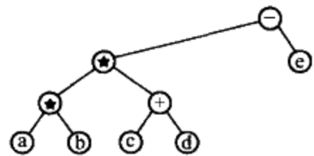
图 4-70 练习 4.8 中的树
