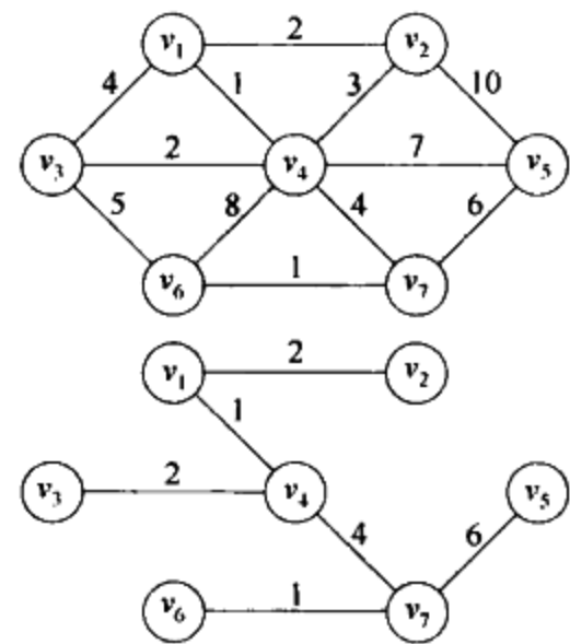
图 9-48 图 G 及其最小生成树
