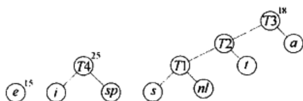
图 10-17 第四次合并后的哈夫曼算法
