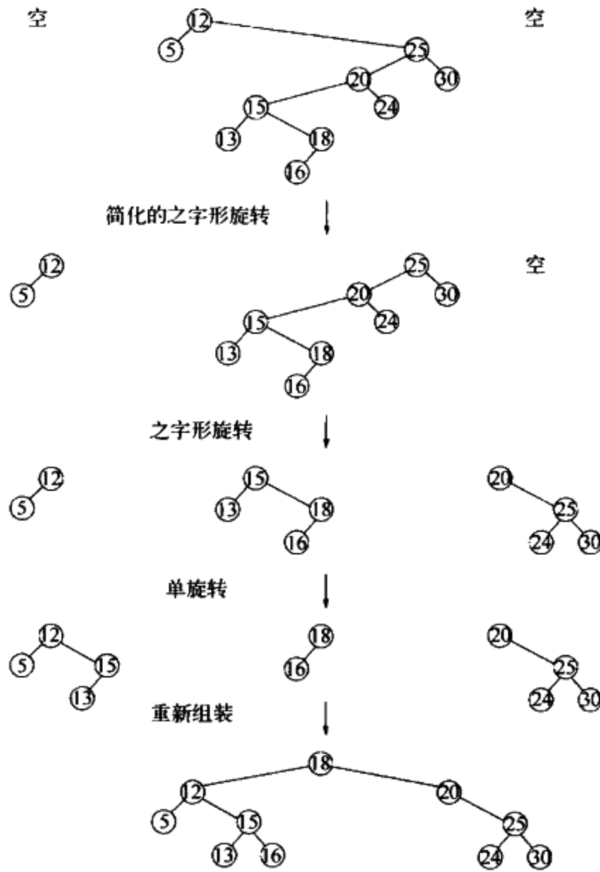
图 12-4 (访问上面树中的 19)自顶向下展开的各步
