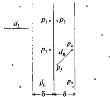
图 10-31 双道带区域,包含对于 d_C 带 所考虑的全部点
