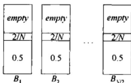
图 10-23 对 0.5, 2/N, 0.5, 2/N, 0.5, 2/N, ... 的下项适合装箱法
