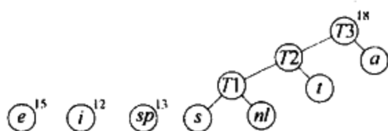
图 10-16 第三次合并后的哈夫曼算法
