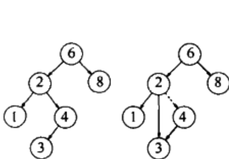
图 4-23 具有一个儿子的节点 4 删除前后的情况
