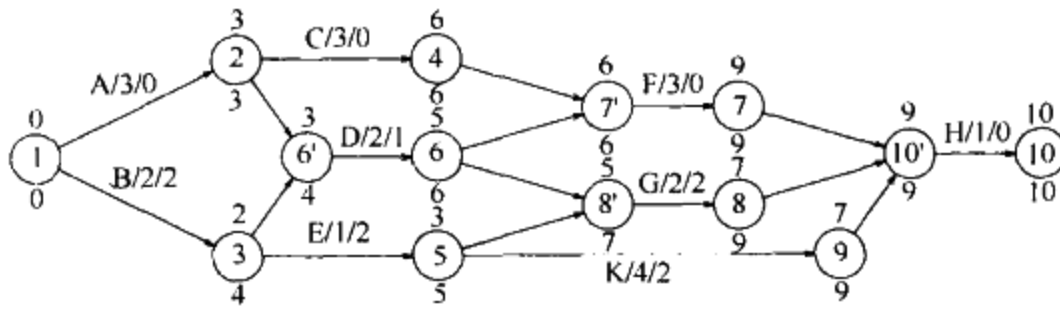
图 9-37 最早完成时间、最晚完成时间和松弛时间
