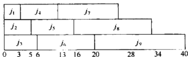
图 10-5 多处理器情形的一个最优解
