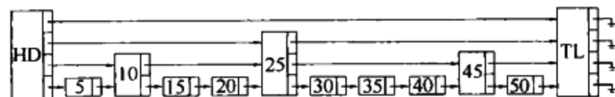
图 12-19 插入 27：首先，通过提升 25 将含 3 个高度为 2 的节点的间隙分裂
