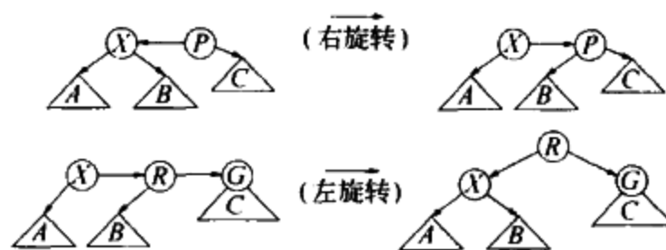
图 12-30 skew 和 split。注意 R 的层次在一次 split 中增加
