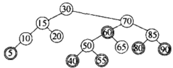
图 12-9 红黑树的例子(插入序列为: 10, 85, 15, 70, 20, 60, 30, 50, 65, 80, 90, 40, 5, 55)
