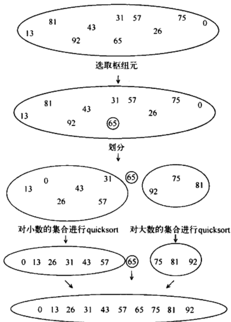
图 7-11 以例说明快速排序的各步
