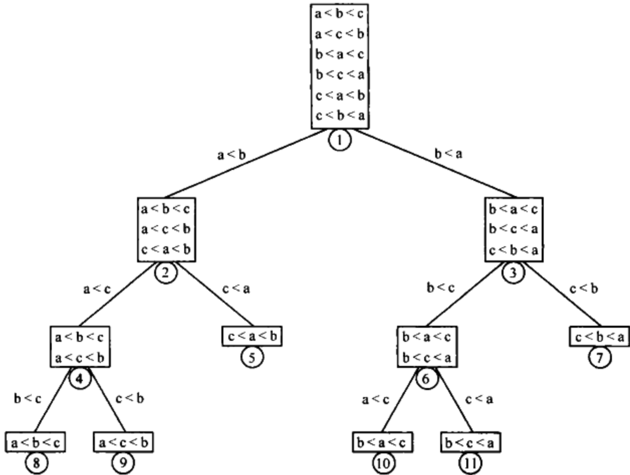
图 7-17 三元素排序的决策树
