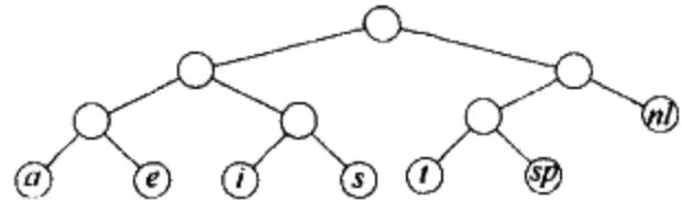
图 10-10 稍微好一些的树
