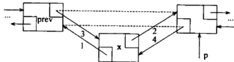
图 3-27 通过获取一个新节点,然后按所指示的顺序改变指针而完成向一个双链表中的插入操作
