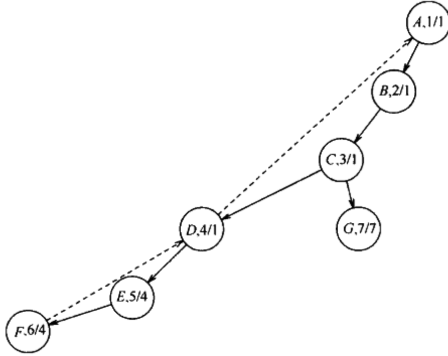
图 9-63 上图的深度优先树，节点标有 Num 和 Low
