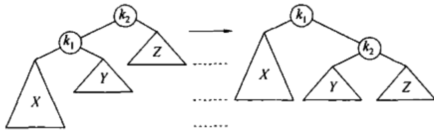
图 4-31 调整情形 1 的单旋转
