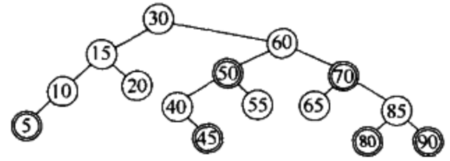
图 12-12 将 45 插入到图 12-9 中
