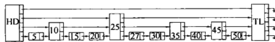
图 12-21 插入 27：最后，将 27 作为高度为 1 的节点插入
