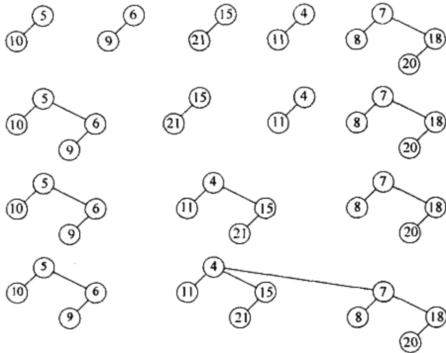
图 11-18 把一些二项树合并成一个二项队列
