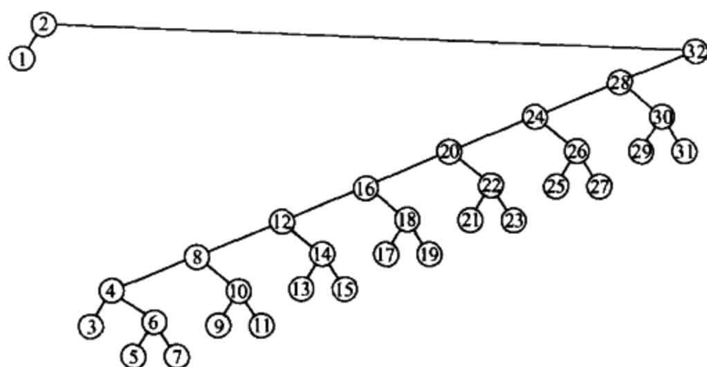
图 4-48 将前面的树在节点 2 展开的结果
