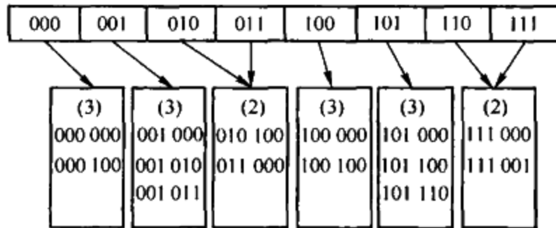
图 5-26 可扩散列: 在 000 000 插入及树叶分裂后
