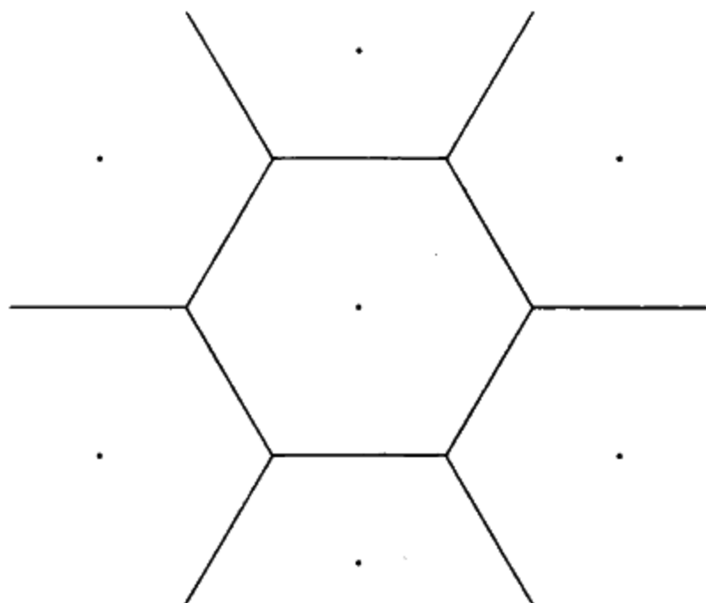
图 10-77 Voronoi 图
