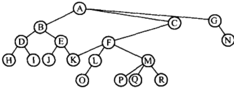
图 4-72 练习 4.44 中的树
