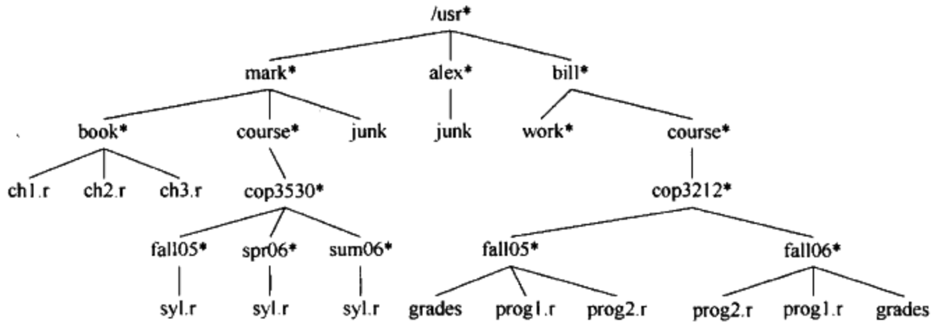
图 4-5 UNIX 目录
