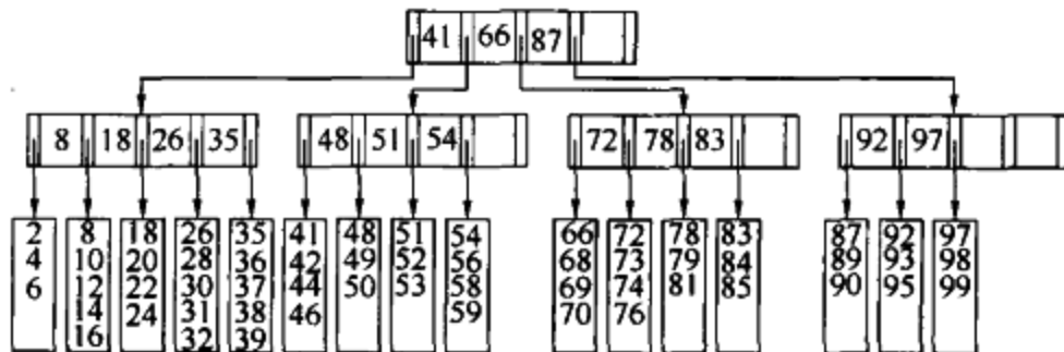
图 4-59 5 阶 B 树
