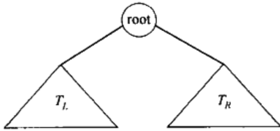
图 4-11 一般二叉树
