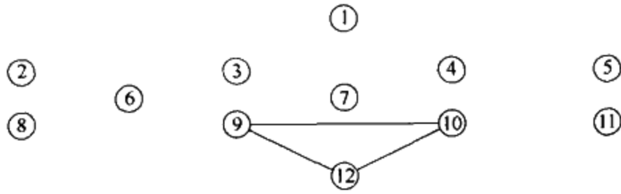
图 9-73 在路径 5,4,1,3,2,8,9,6,3,7,4,11,10,7,9,3,4,10,5 后剩下的图
