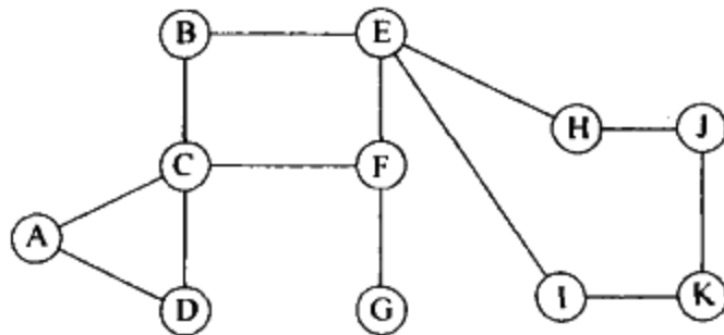
图 9-83 练习 9.21 中的图
