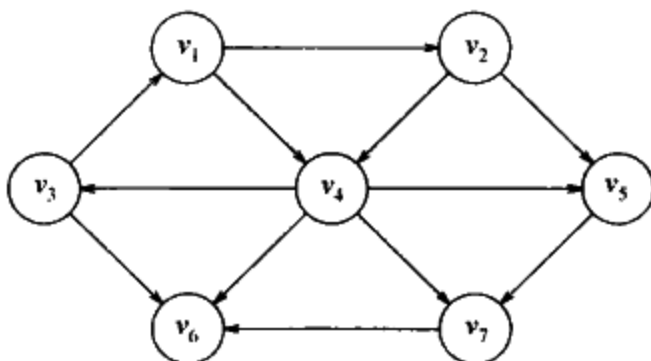
图 9-10 一个无权有向图 G
