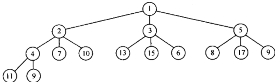
图 6-19 一个 d -堆
