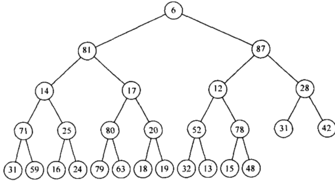
图 6-57 最小-最大堆
