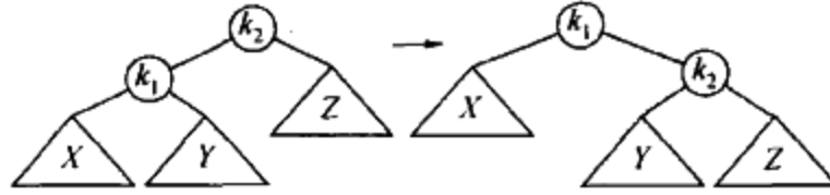
图 4-40 单旋转
