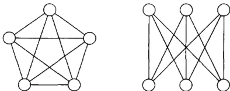
图 9-85 练习 9.35 中使用的图
