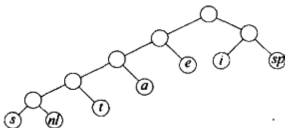
图 10-11 最优前缀码
