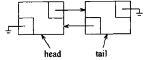
图 3-23 具有头节点和尾节点的空链表
