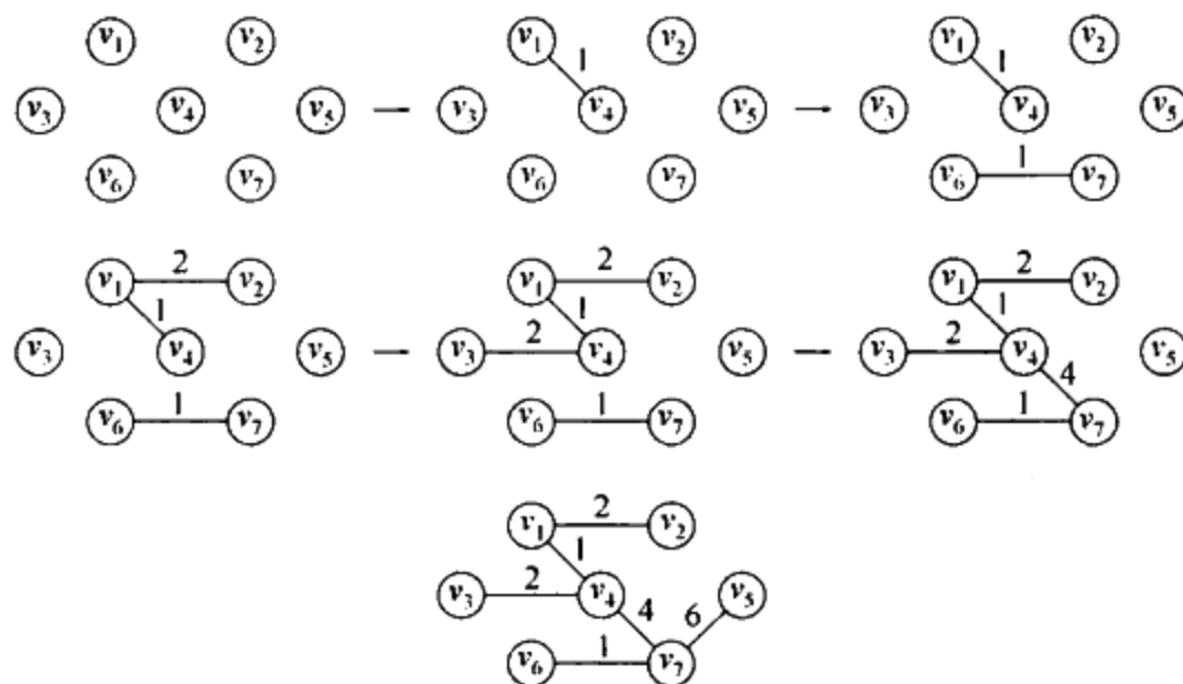
图 9-57 在每一步之后的 Kruskal 算法
