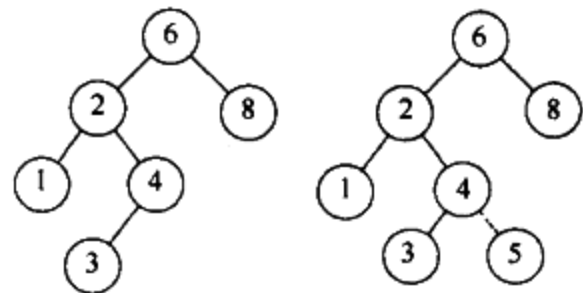
图 4-21 在插入 5 以前和以后的二叉查找树
