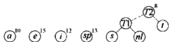
图 10-15 第二次合并后的哈夫曼算法
