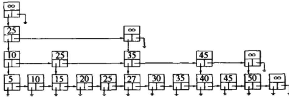
图 12-22 图 12-21 中 1-2-3 确定性跳跃表的链表实现
