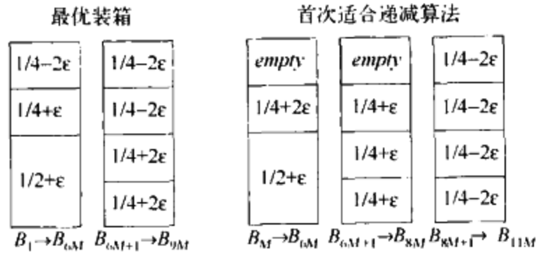
图 10-28 首次适合递减算法使用 11M 个箱子但只有 9M 个箱子就足够完成装箱
