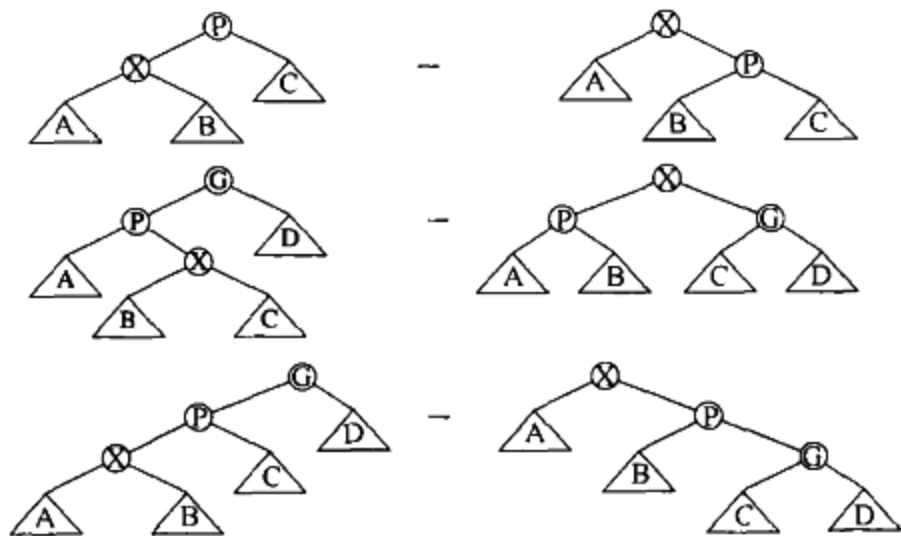
图 11-21 单旋转、之字形和一字形双旋转操作;每个都有一个对称的情形(未示出)
