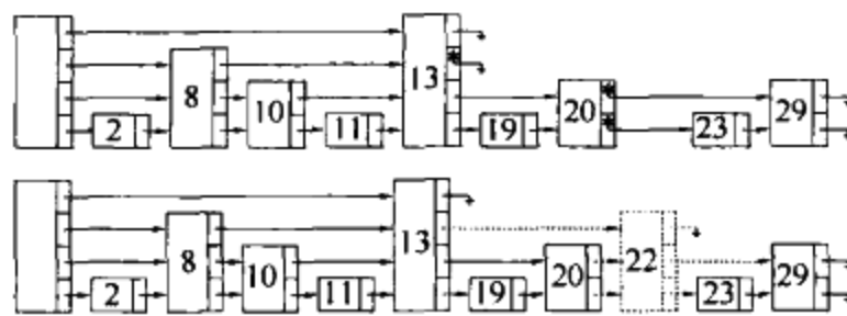
图 10-61 插入前和插入后的跳跃表
