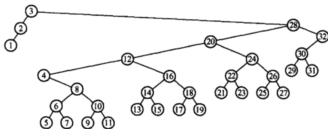
图 4-49 将前面的树在节点 3 处展开
