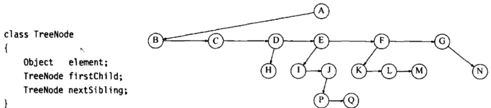
图 4-3 树节点的声明
