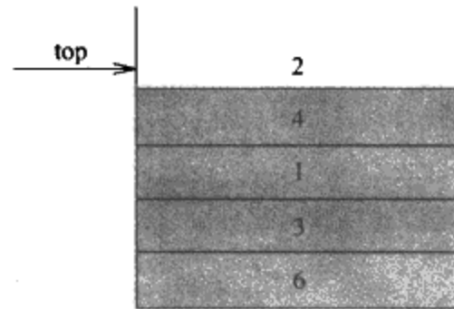
图 3-34 栈模型：只有栈顶元素是可访问的
