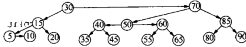
图 12-32 在 35 处进行 split 之后
