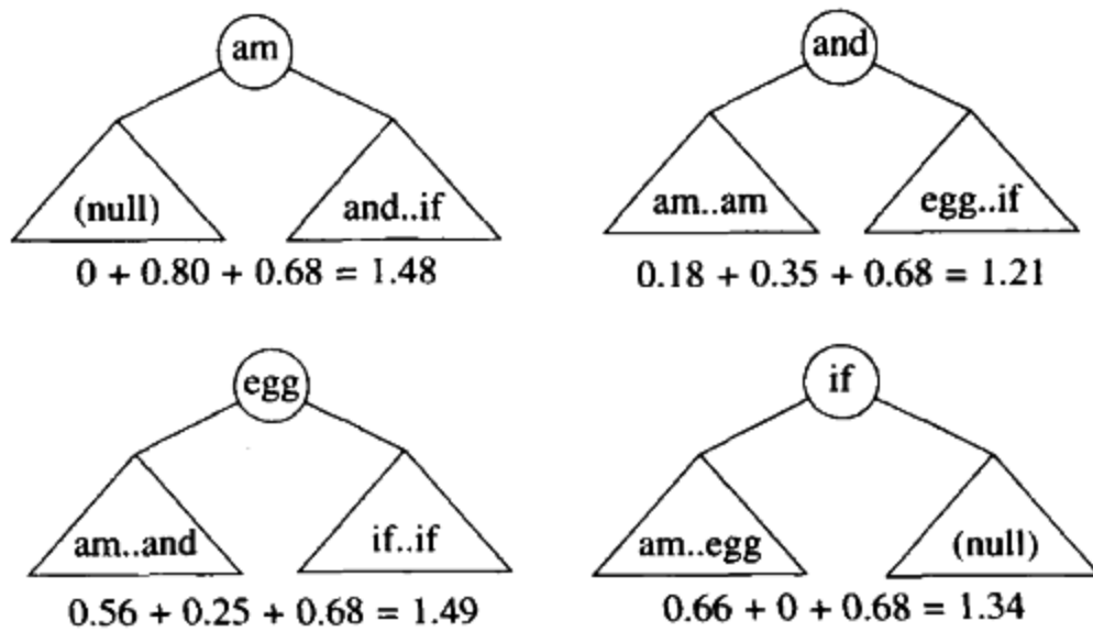
图 10-52 对 am..if 的表项(1.21, and)的计算
