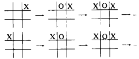
图 10-68 到达同一位置的两种搜索
