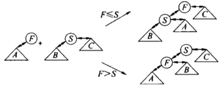
图 12-47 compareAndLink 合并两个子堆
