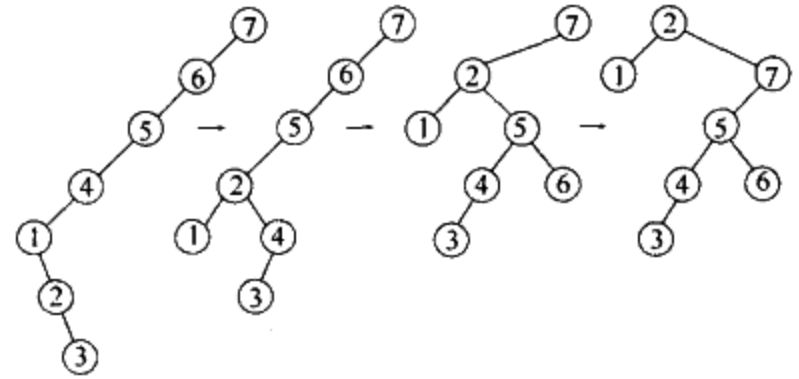
图 11-22 在节点 2 展开中涉及的展开各步
