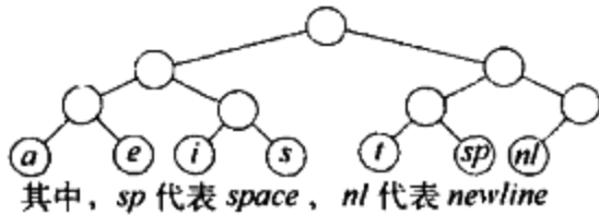
图 10-9 树中原始代码的表示法
