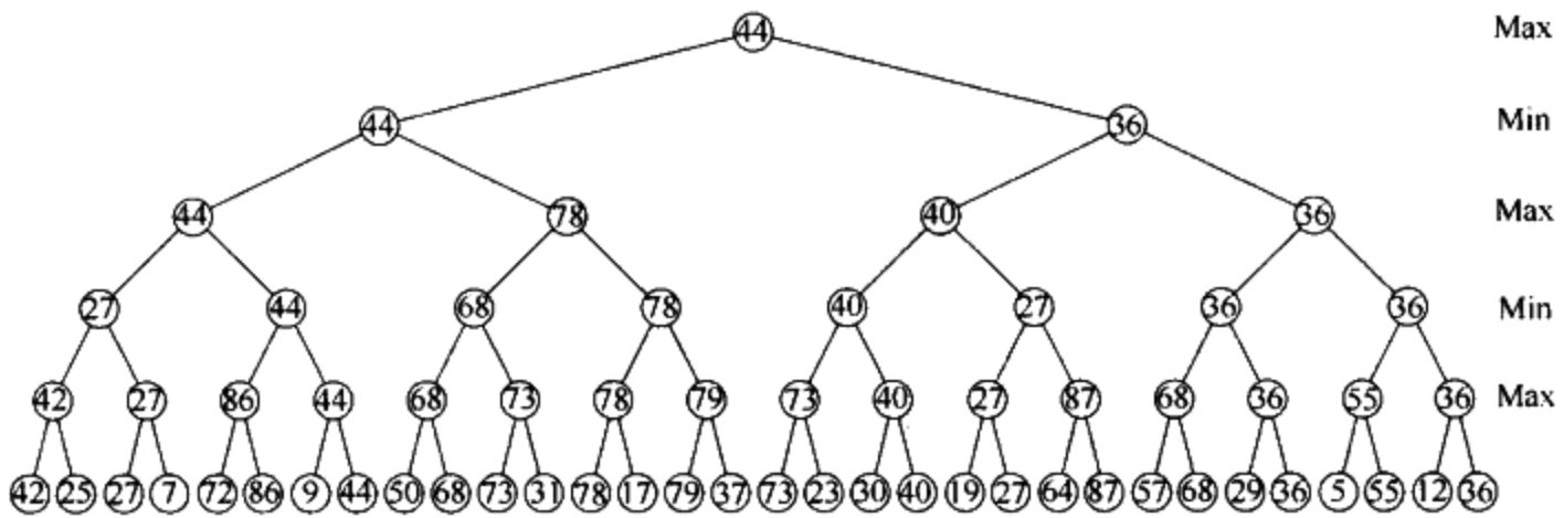
图 10-69 一棵假想的博弈树
