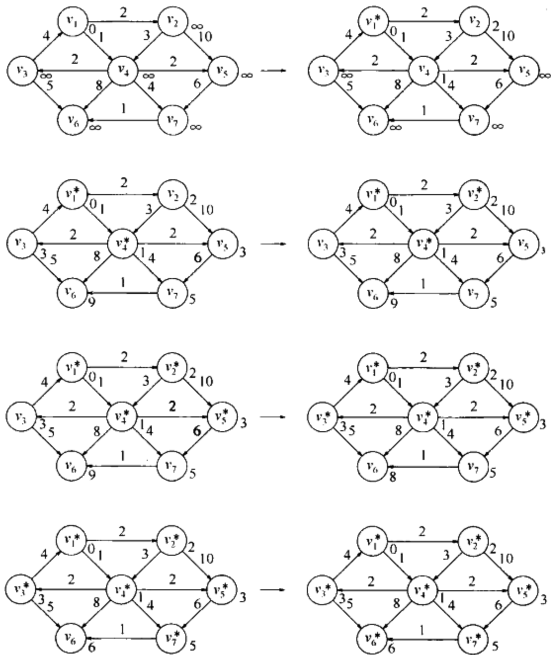
图 9-28 Dijkstra 算法的各个阶段
