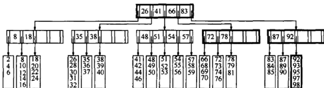
图 4-63 在从图 4-62 的 B 树中删除 99 后的 B 树
