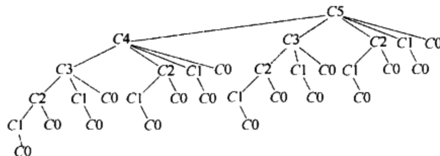
图 10-44 跟踪方法 eval 中的递归计算
