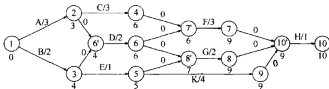
图 9-36 最晚完成时间
