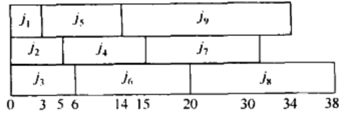
图 10-6 多处理器情形的第二个最优解
