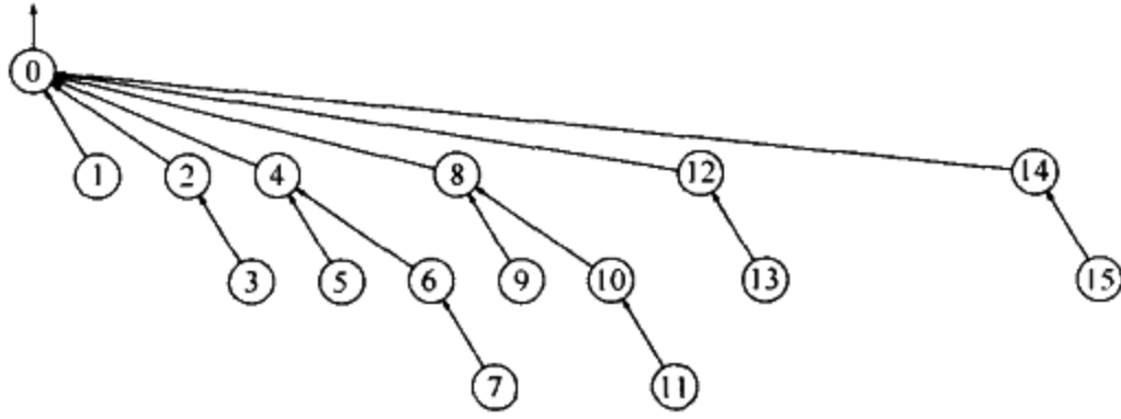
图 8-14 路径压缩的一个例子
