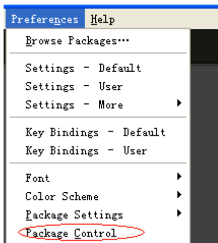
图1.7 sublime包管理
