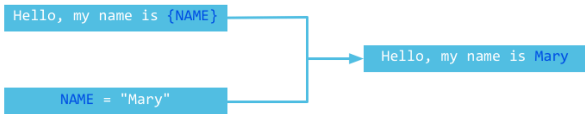
图7.1 模板机制图
