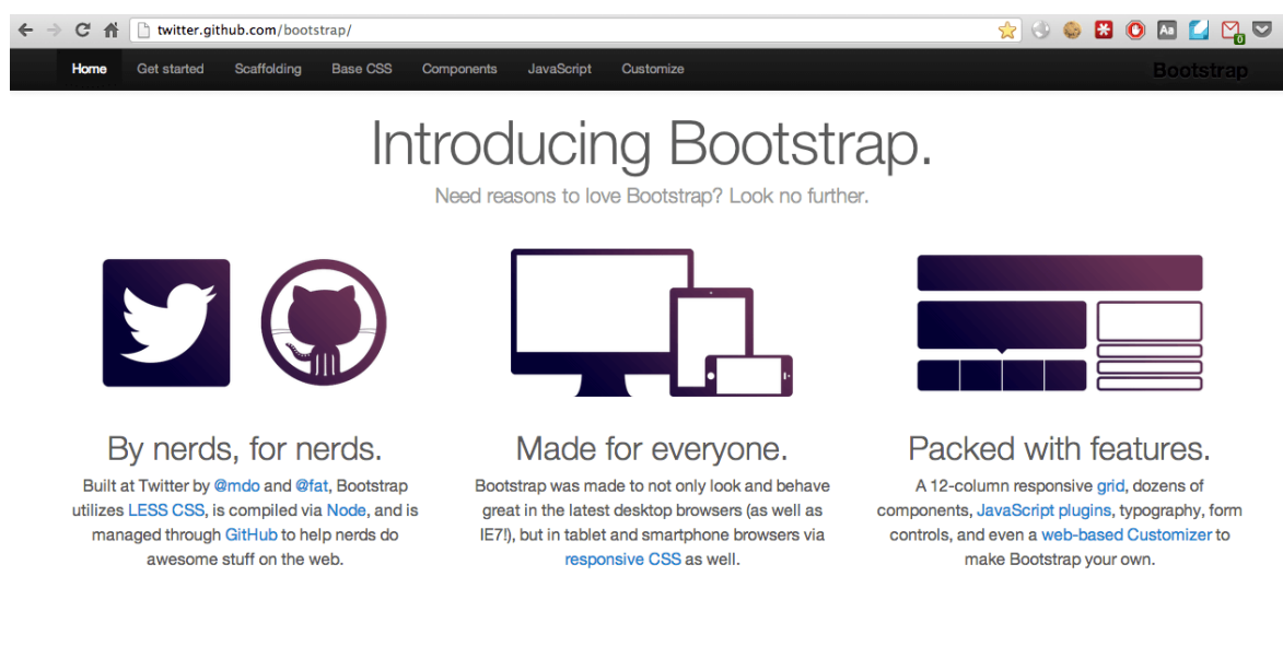
图14.1 bootstrap站点
