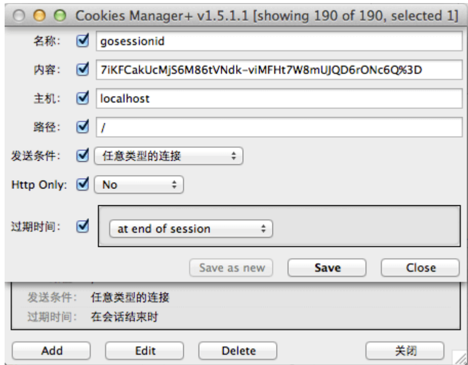
图6.6 模拟cookie
