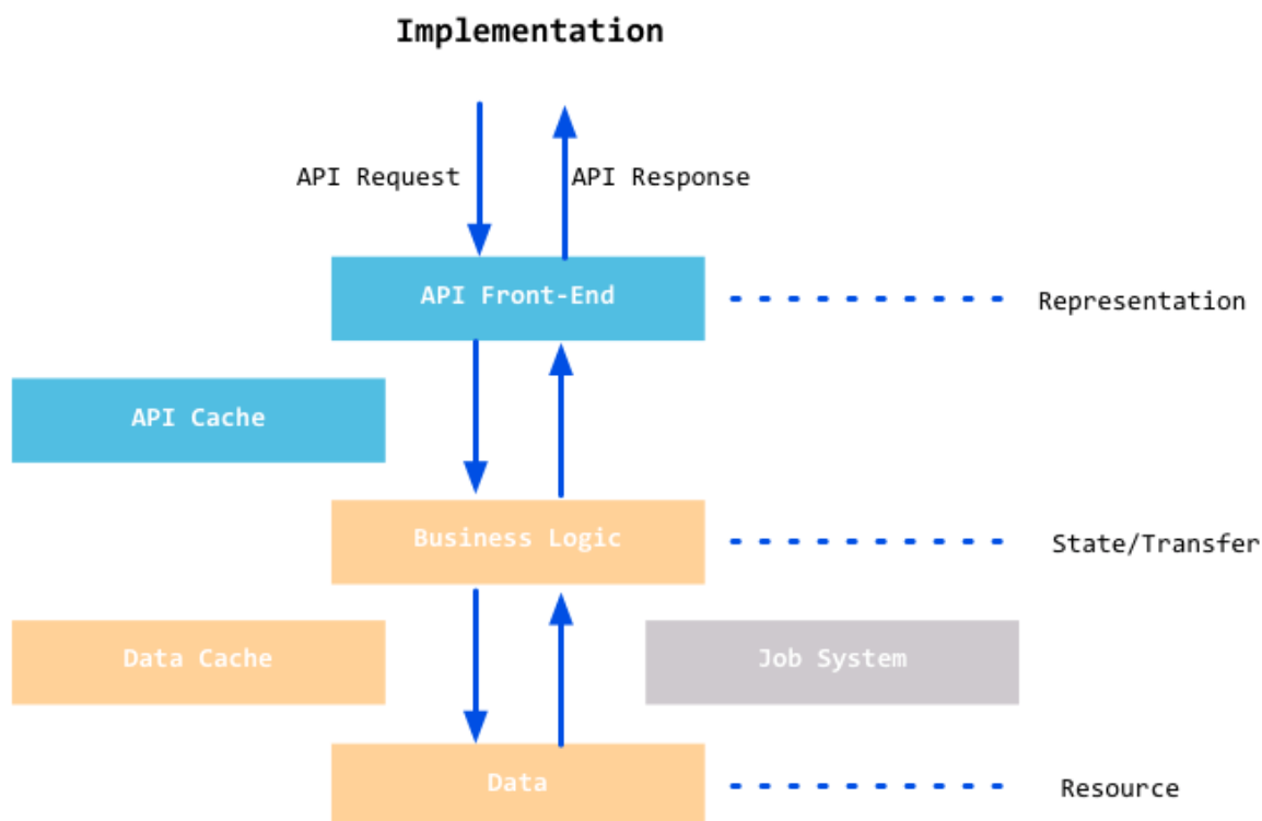
图8.5 REST架构图
