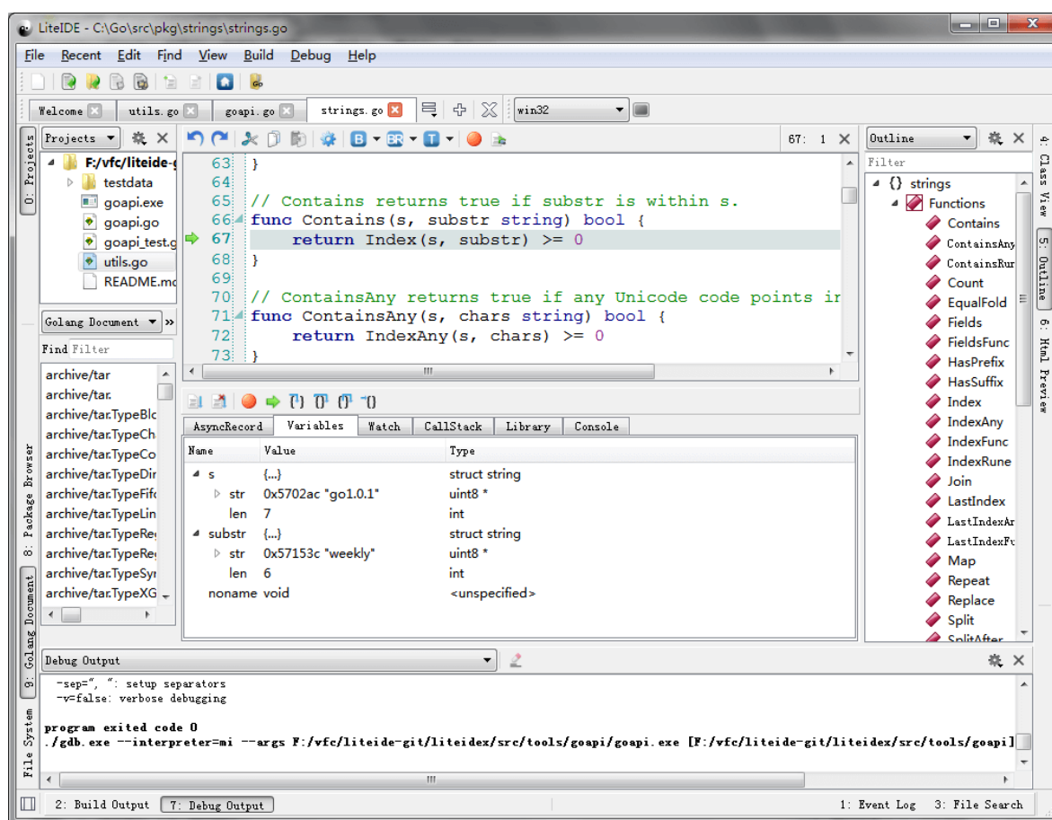
图1.4 LiteIDE主界面
