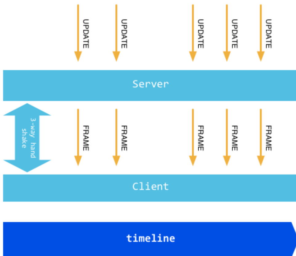
图8.2 WebSocket原理图
