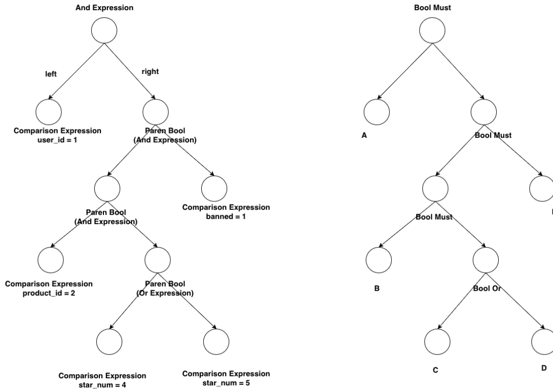
图 6-12 AST和DSL之间的对应关系
