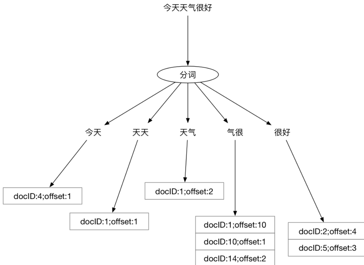
图 6-11 “今天天气很好”的分词结果
