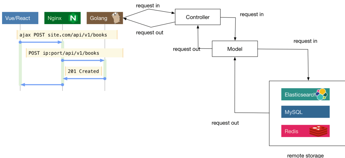
图 5-13 前后分离交互图
