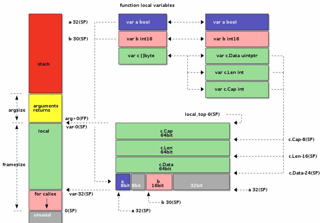
图 3-11 函数的局部变量
