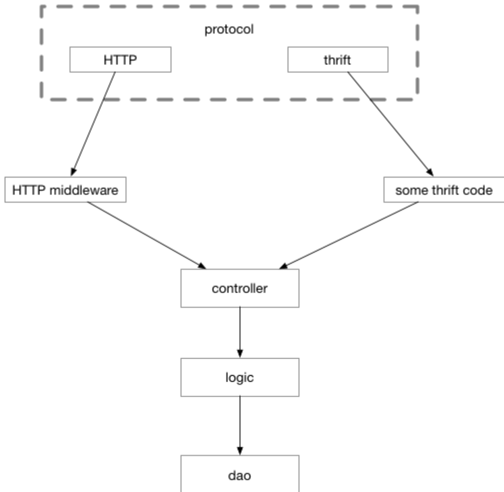
图 5-18 加入中间件后的控制流
