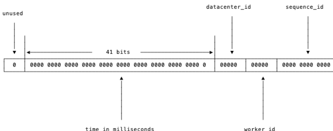
图 6-1 snowflake 中的比特位分布
