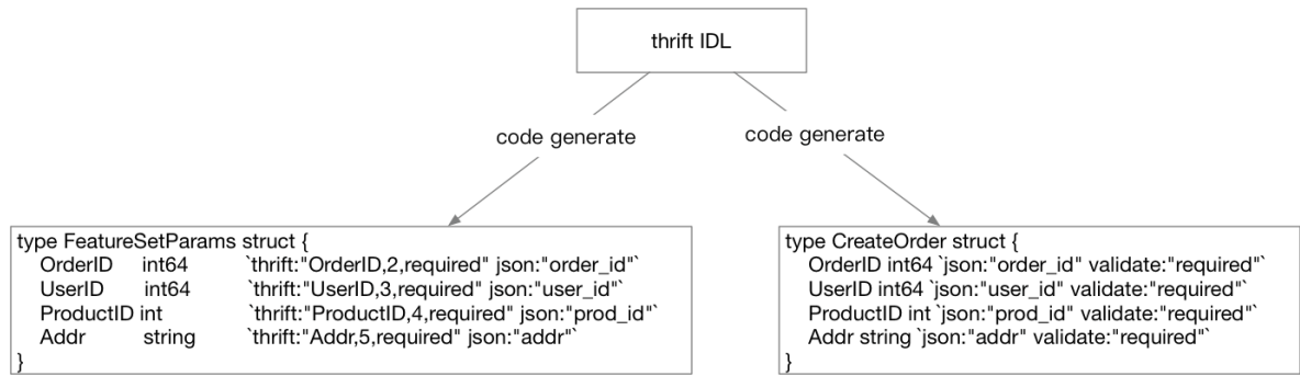
图 5-17 也可以从thrift生成其它部分
