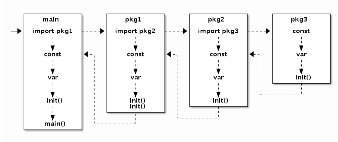
图 1-12 包初始化流程
