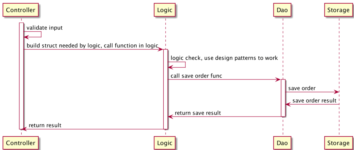
图 5-14 请求处理流程
