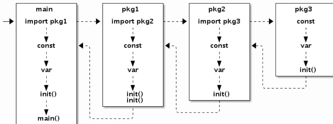
图 1-11 包初始化流程
