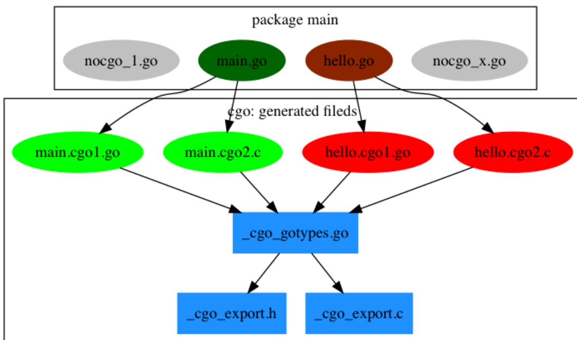
图 2-4 cgo生成的中间文件
