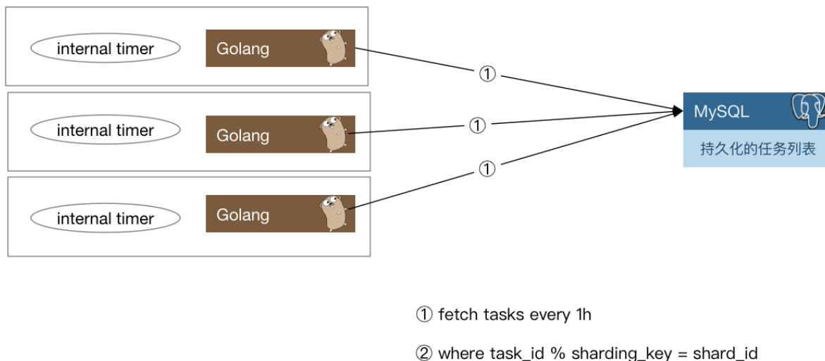
图 6-7 分布式任务分发
