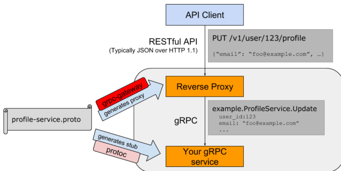
图 4-2 gRPC-Gateway 工作流程
