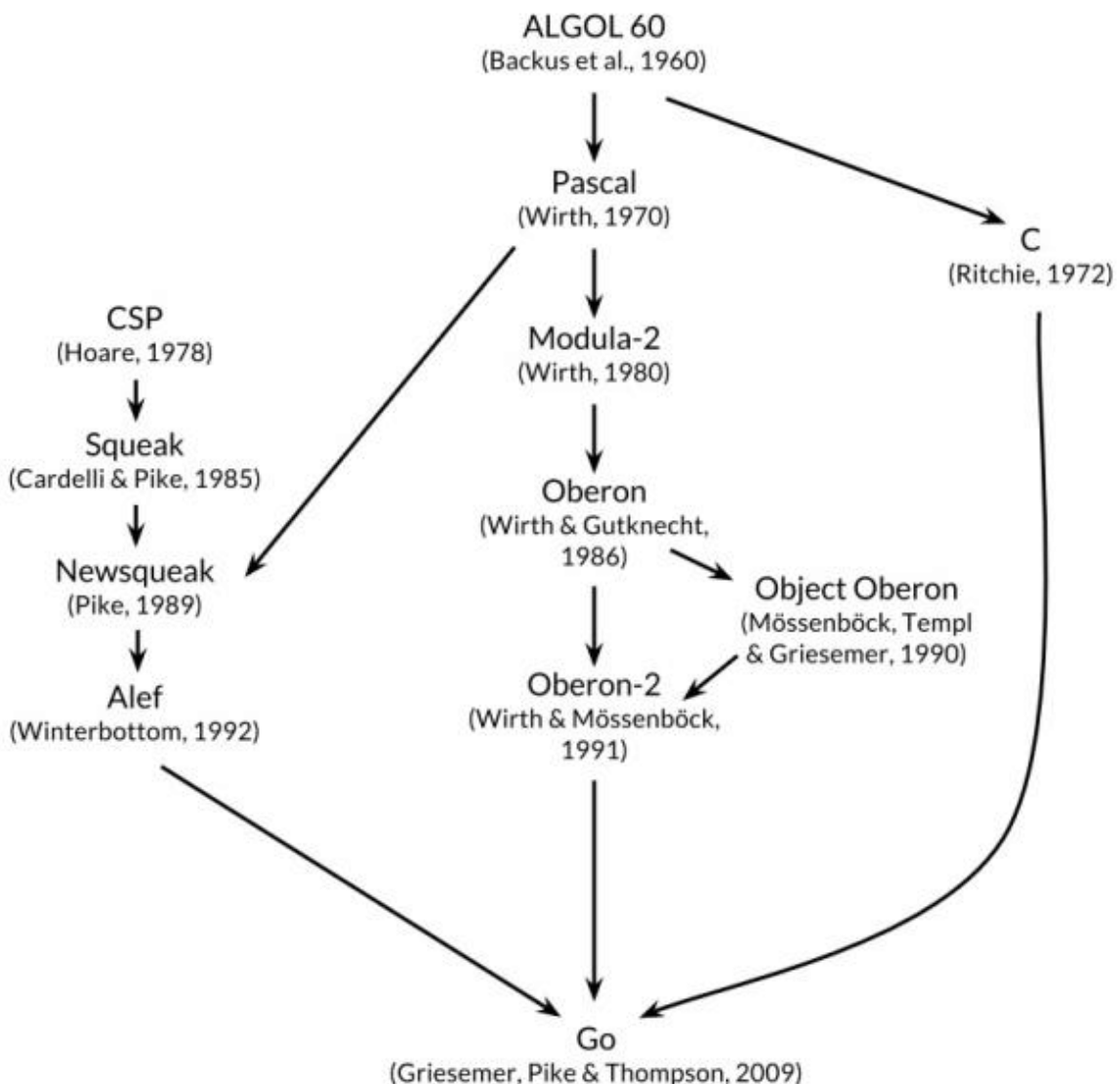
图 1-1 Go 语言基因族谱
