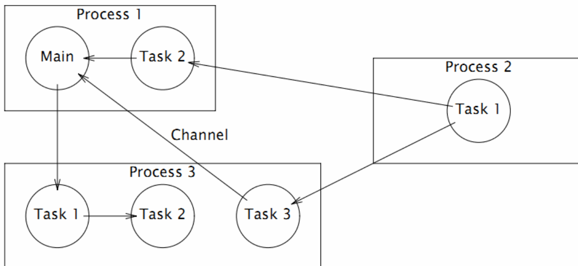
图 1-6 Alef并发模型
