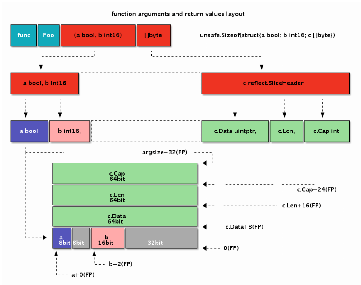
图 3-10 函数的参数
