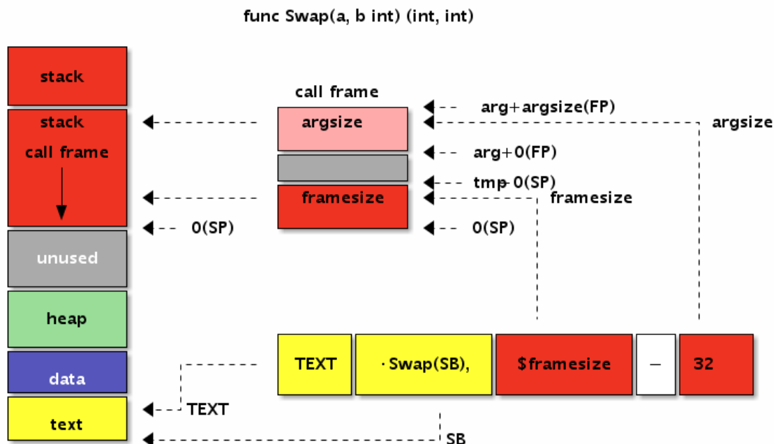
图 3-9 函数定义
