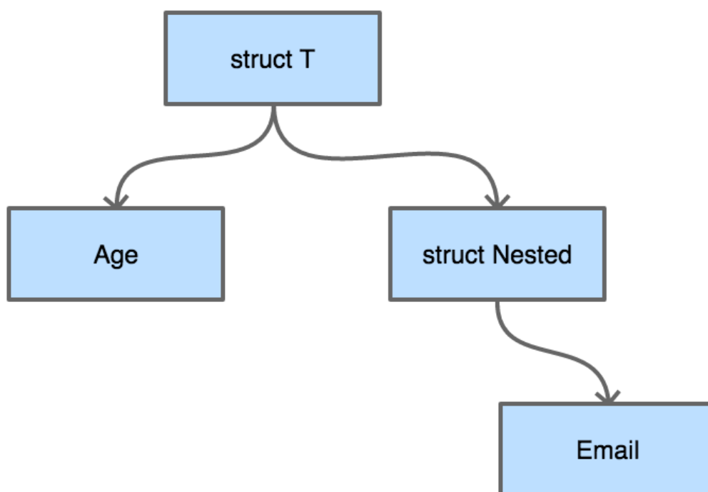
图 5-11 validator 树
