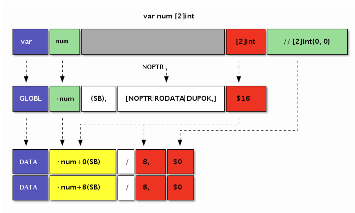
图 3-4 变量定义
