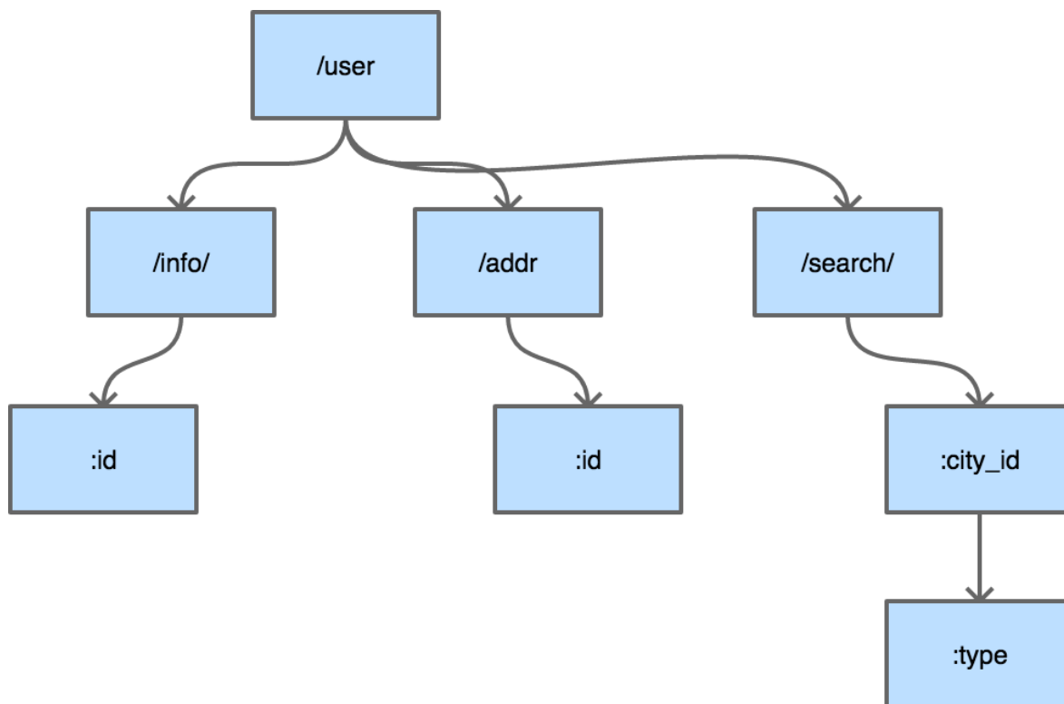
图 5-2 压缩字典树
