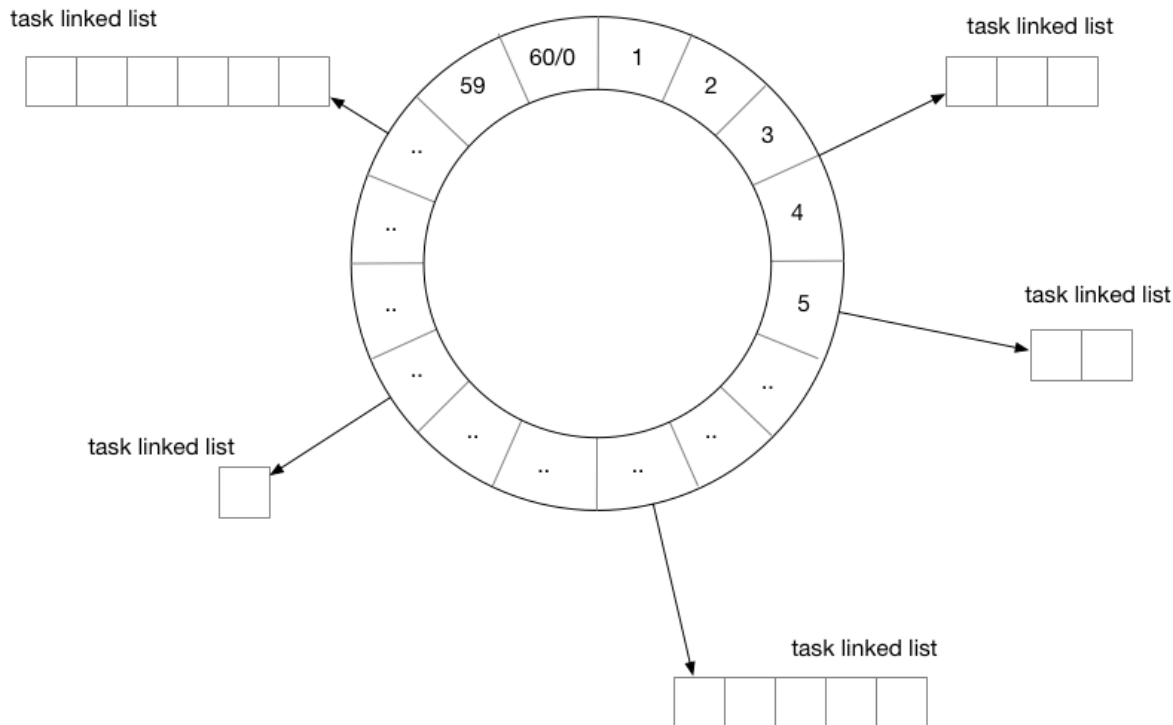
图 6-6 时间轮
