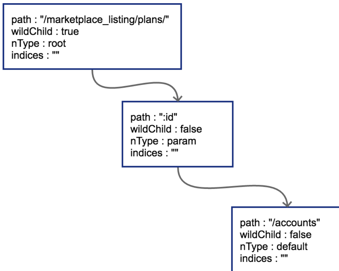
图 5-5 插入第二个节点的压缩字典树
