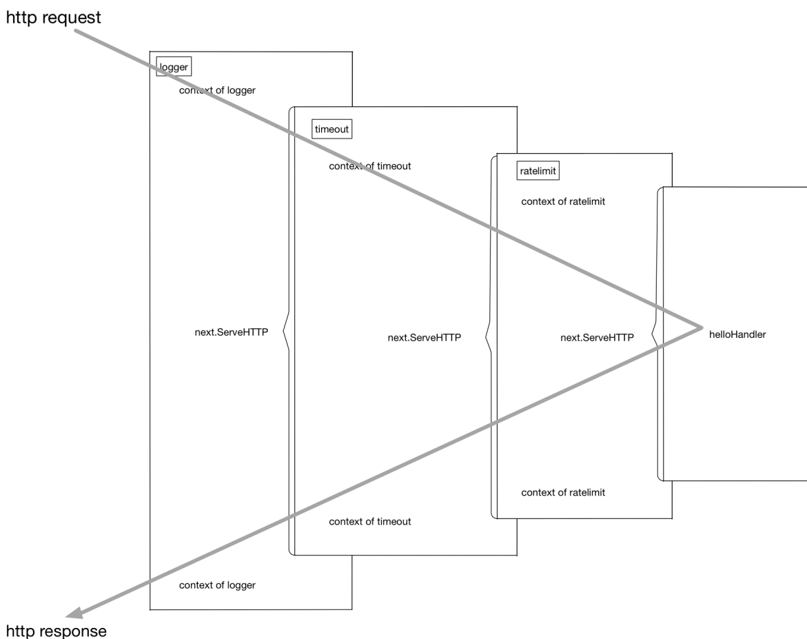
图 5-8 请求处理过程
