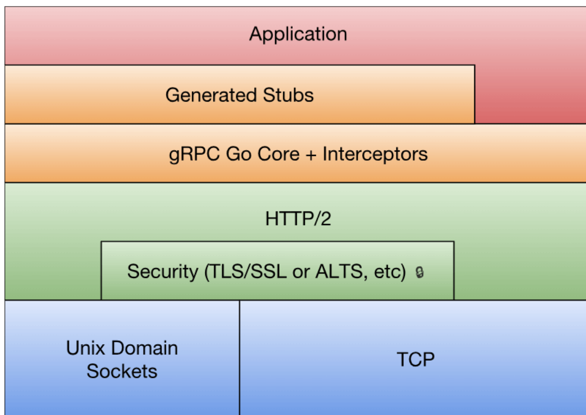
图4-1 gRPC技术栈
