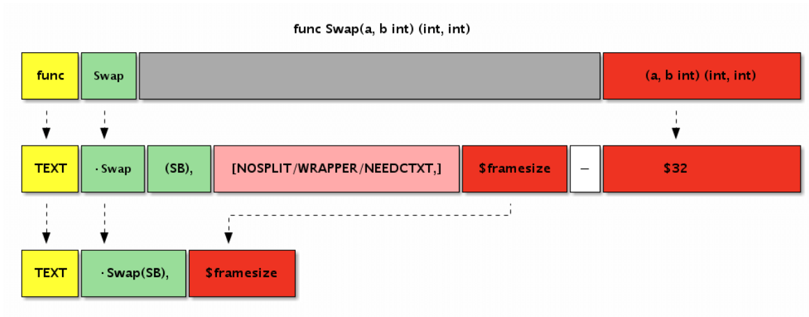
图 3-8 函数定义
