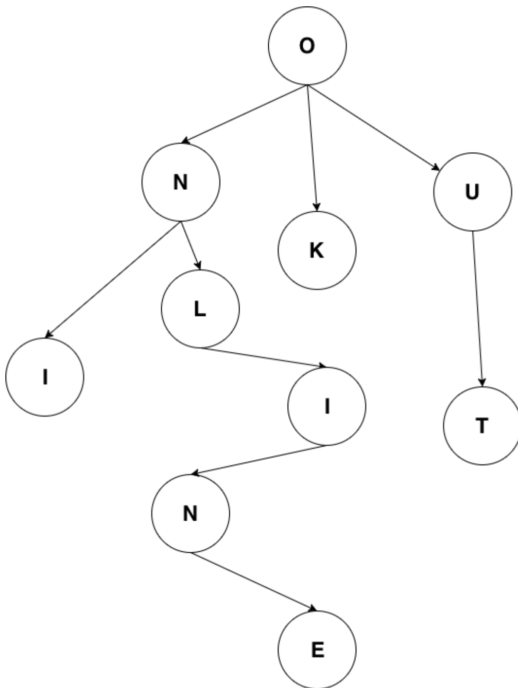
图 5-1 字典树
