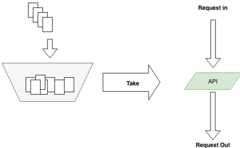
图 5-12 令牌桶
