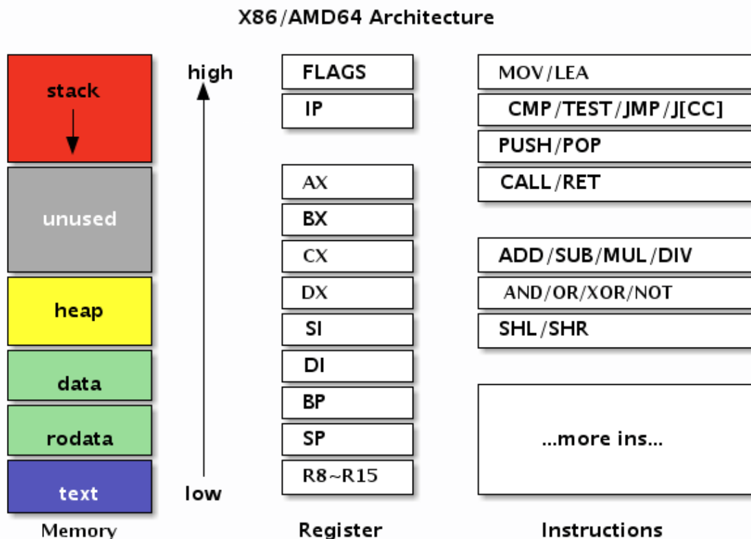
图 3-2 AMD64 架构
