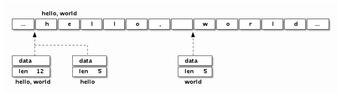
图 1-8 字符串布局
