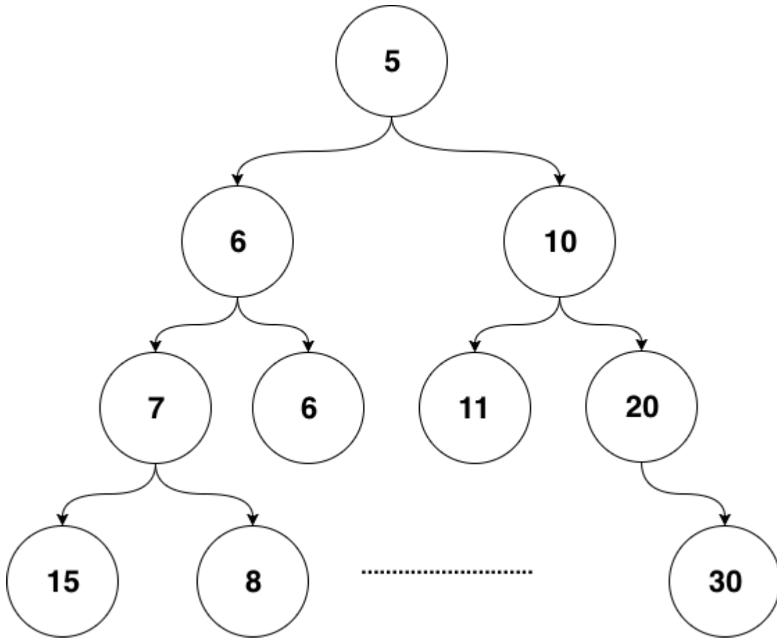
图 6-4 二叉堆结构
