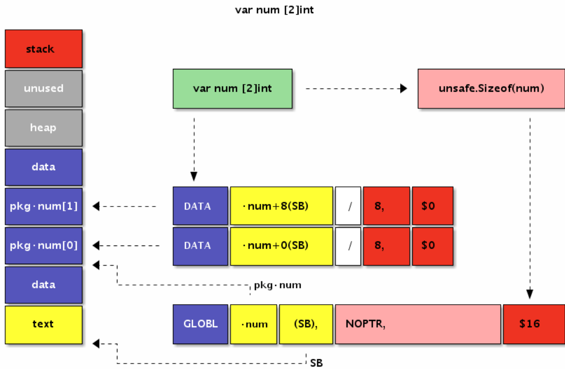
图 3-6 变量定义
