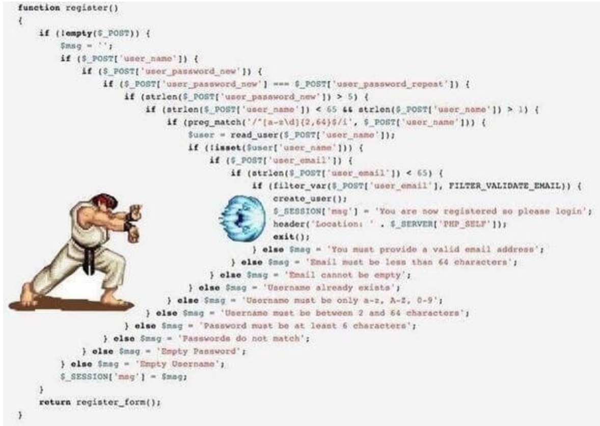
图 5-10 validator 流程
