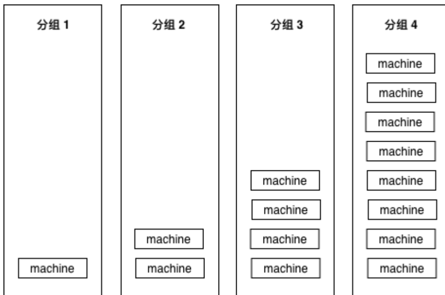
图 5-20 分组部署
