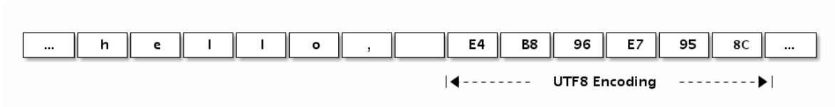
图 1-9 字符串布局
