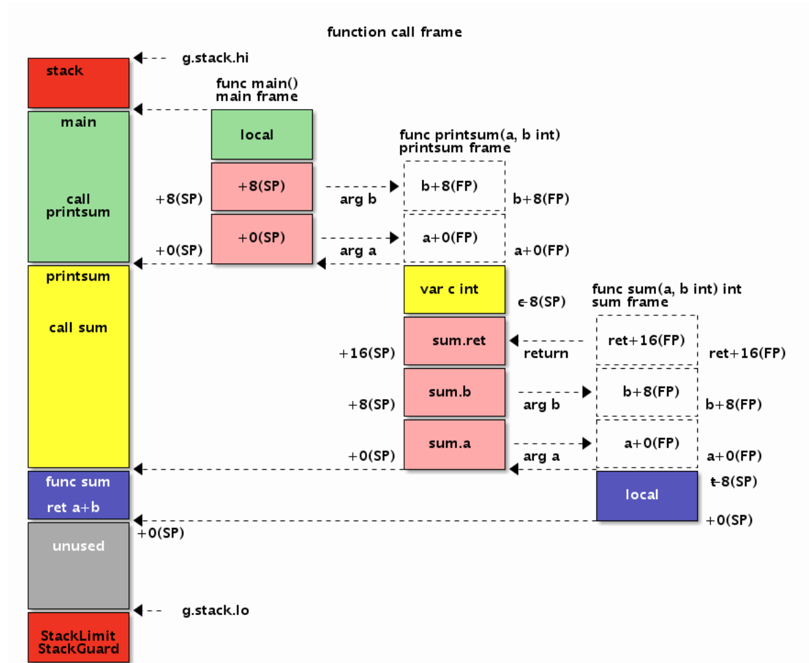
图 3-12 函数帧
