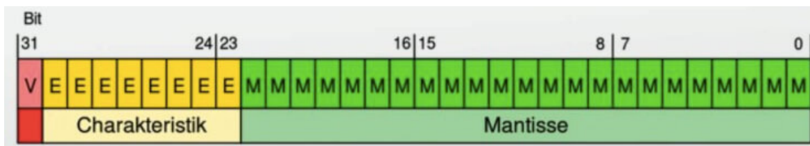
图 3-5 IEEE754浮点数结构
